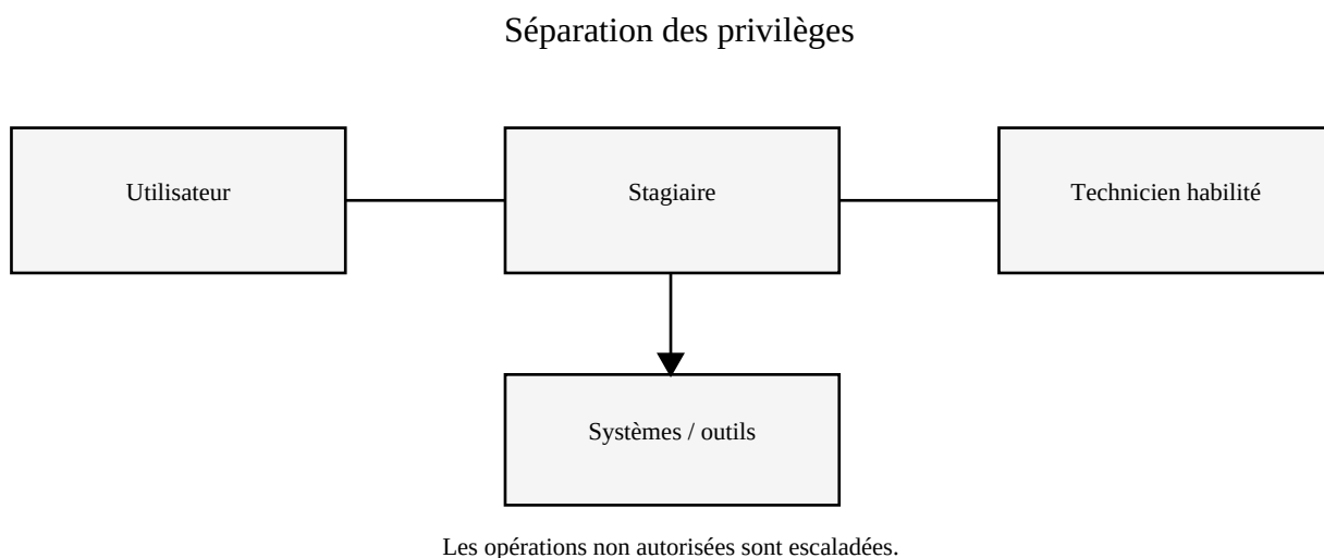
Figure 9 — Principe de séparation des privilèges.
